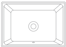
Art. 8032 - 56 x 39,5 x h1,5 cm / total 15,5 cm GAIA 50
