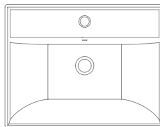
rt. 3004 - 61,5 x 47 x h5 cm / total 16,5 cm ML 60 x 47
