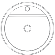
Art. 8055/R - Ø46 x h30 cm MATTY TONDO R
