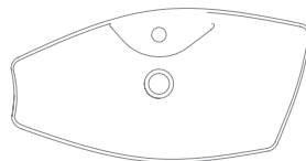
Art. 8052/R - 72 x 37 x h13 cm KONG 70R
