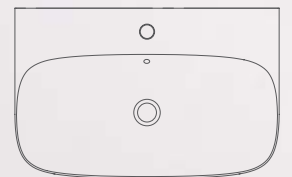
Art. 5508 - 70 x 45 x h15 cm MOON 70R H15
