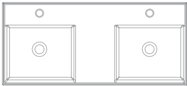
Art. 5142 - 101 x 46 x h14 cm TEOREMA 2.0 101 x 46
