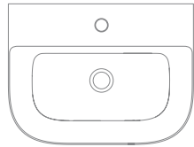
1811 - 55 x 42 x h14 cm GLAM 55/S
