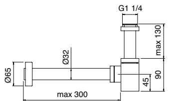
Art. 10009 Sifone tondo in ottone ribassato 1" 1/4 cromato Cp Brass round trap, shorted 1" 1/4 chromed Syphon petit culot laiton chromé Siphon aus verchromtem messing, abgeflacht Sifón redondo de latón rebajado 1" 1/4 cromado Сифон круглого сечения 1" 1/4 укороченный, из хромированной латуни
