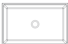
Art. 8031-60 - 60,5 x 38,5 x h13 cm TEOREMA 60
