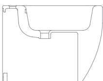
Art. 5139 - 55 x 36 x h42 cm TEOREMA 2.0 BIDET
