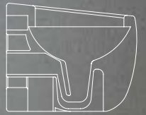
Art. 8401 - 50 x 45 x h44,5 cm PLANET WC
